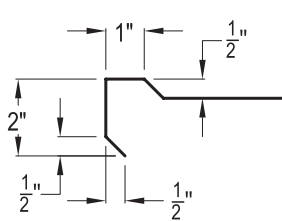
Marine Edge TAC-ME
