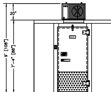
ELEVATION RIGHT HINGE
