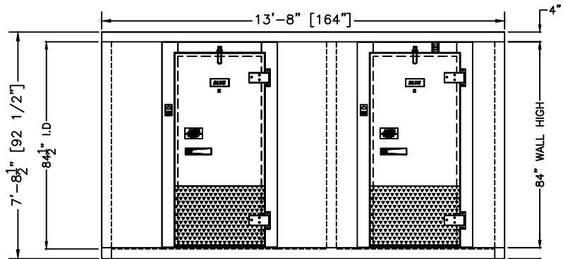
1 ELEVATION SCALE: 1/4"=1'-0"
