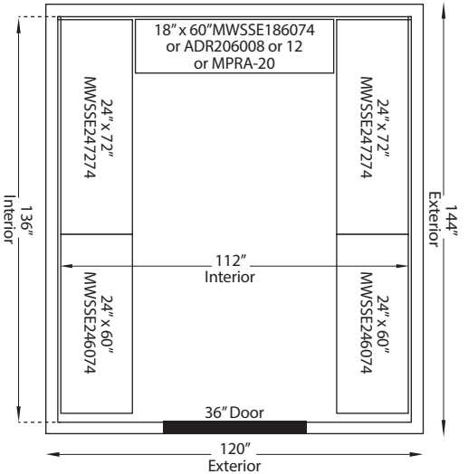
AWC1012-TF-EL/ER
