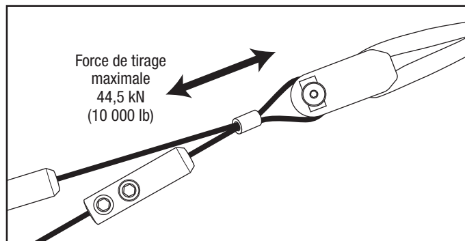
Raccordement typique — Manille et serre-câble
