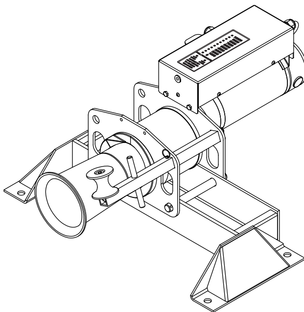
Montaje al piso — Fijado a un piso de concreto
