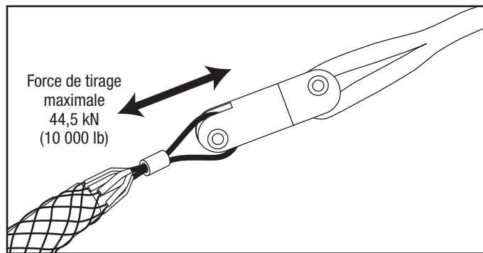
Raccordement typique — Émerillon et tire-câble
