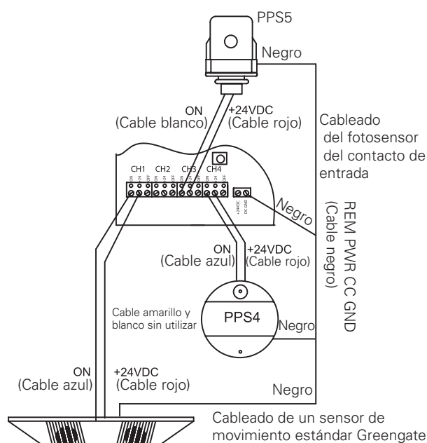
Cableado del sensor de movimiento y de la fotocélula
