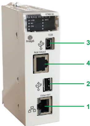
PMXETW0100 Ethway module
